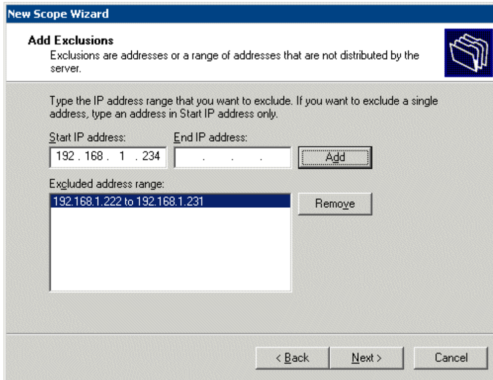
Scope Exclusions
