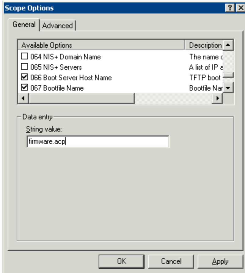
DHCP Options
