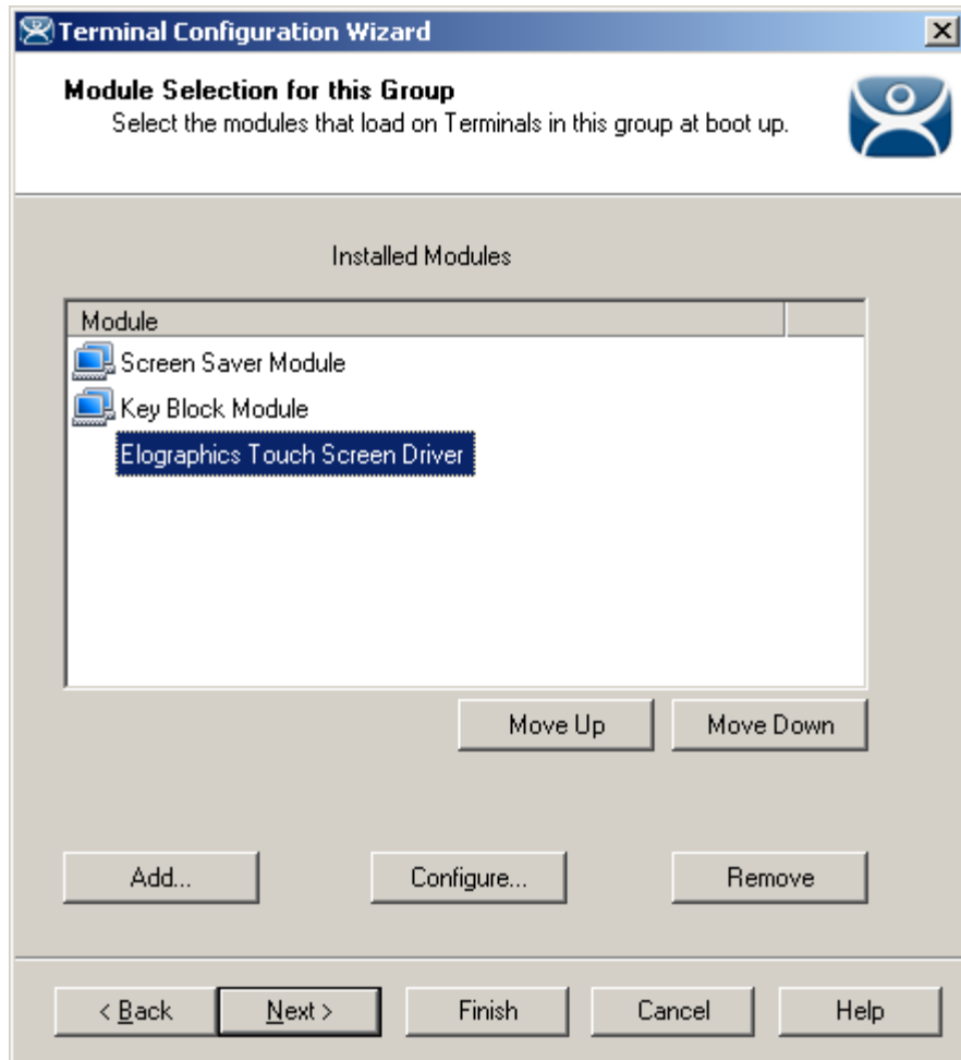
Module Configuration
